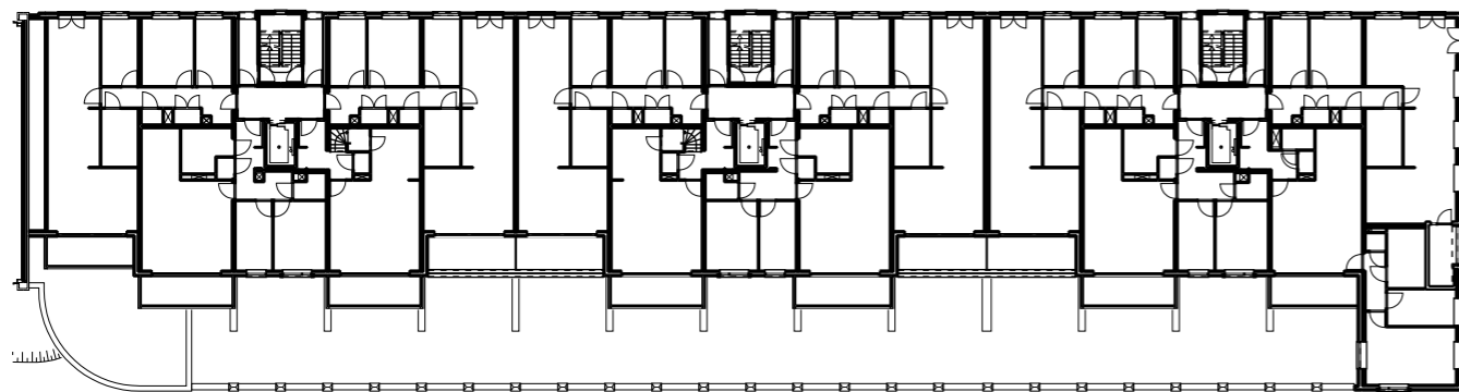
1e verdieping 1:500
