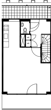
3e verdieping
