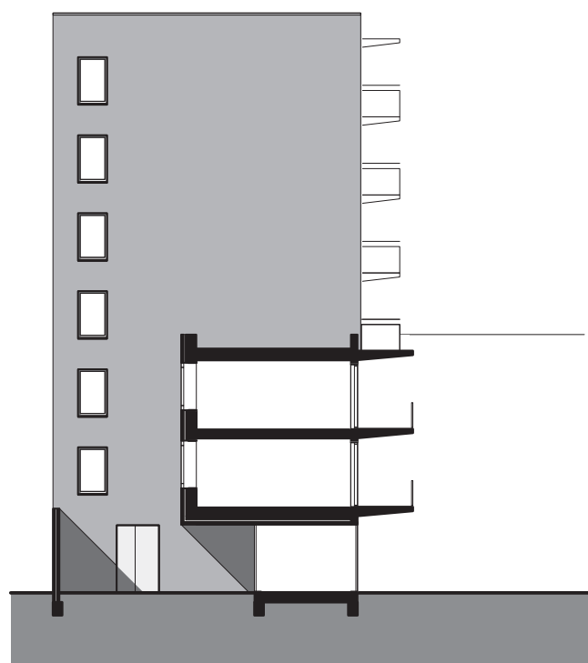
kopgevel toren
