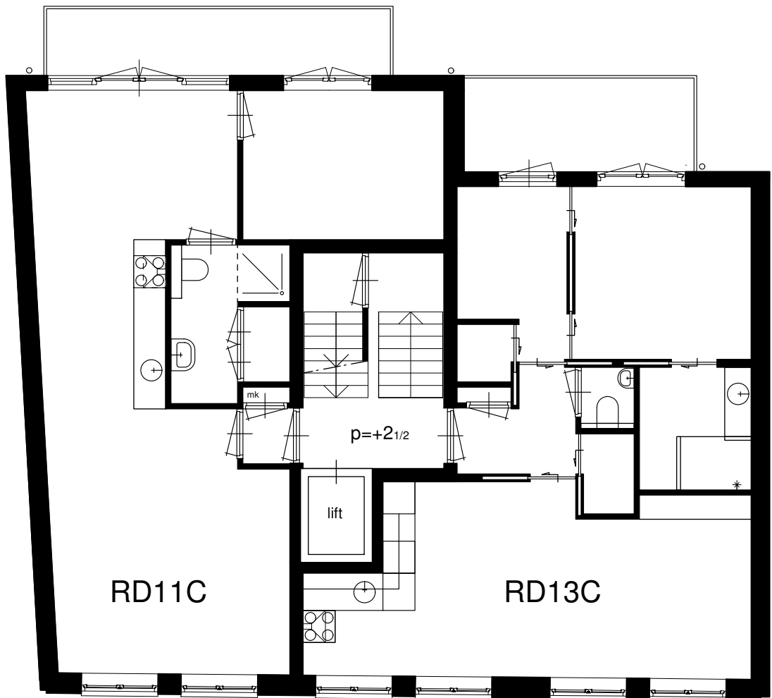
2e verdieping (schaal 1:100)
