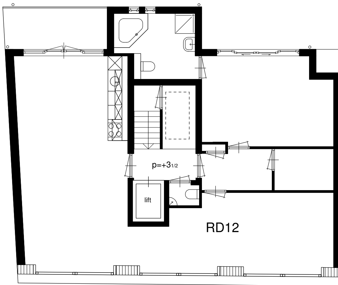
3e verdieping (schaal 1:100)
