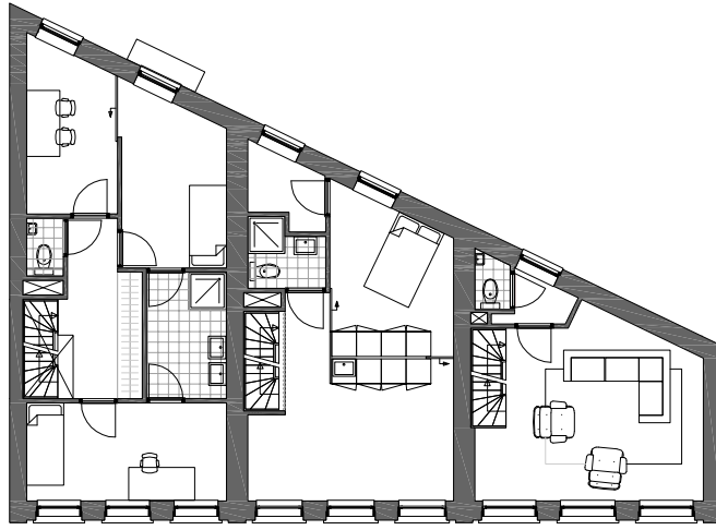
2e verdieping
