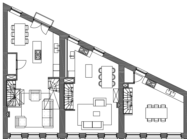
3e verdieping
