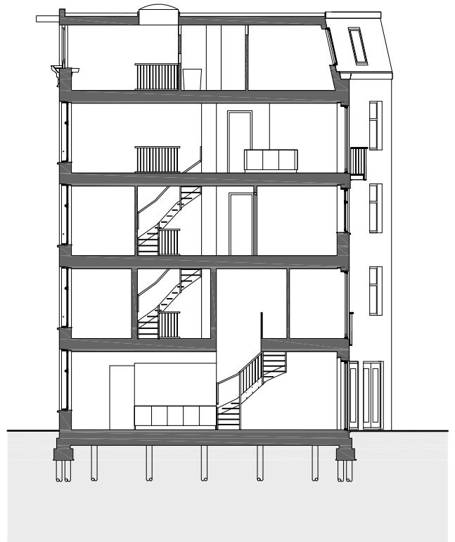
doorsnede
