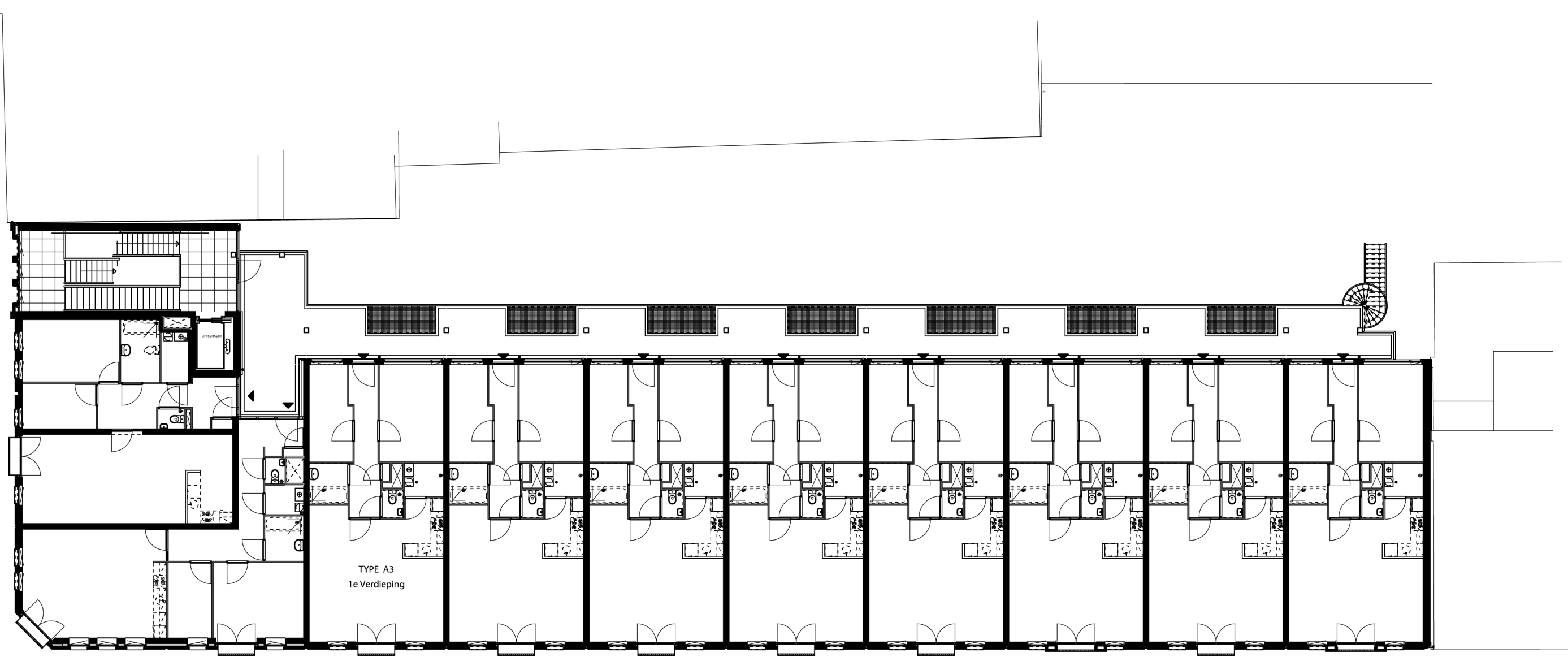
1E VERDIEPING
