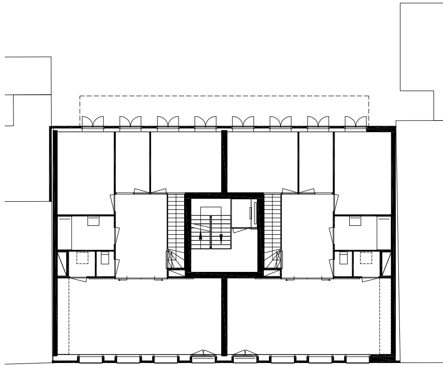
1ste verdieping
