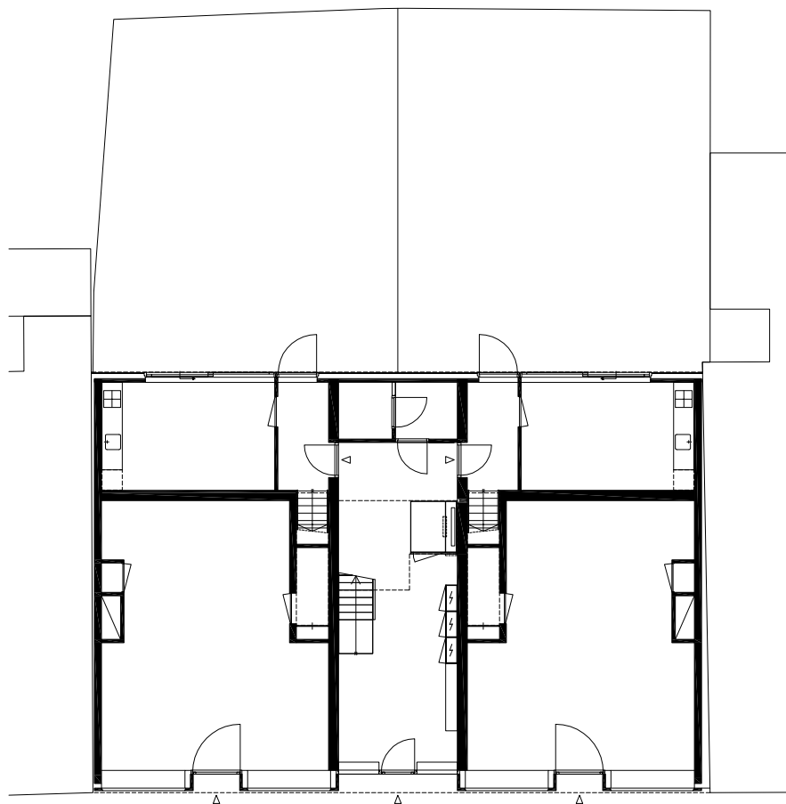
begane grond
