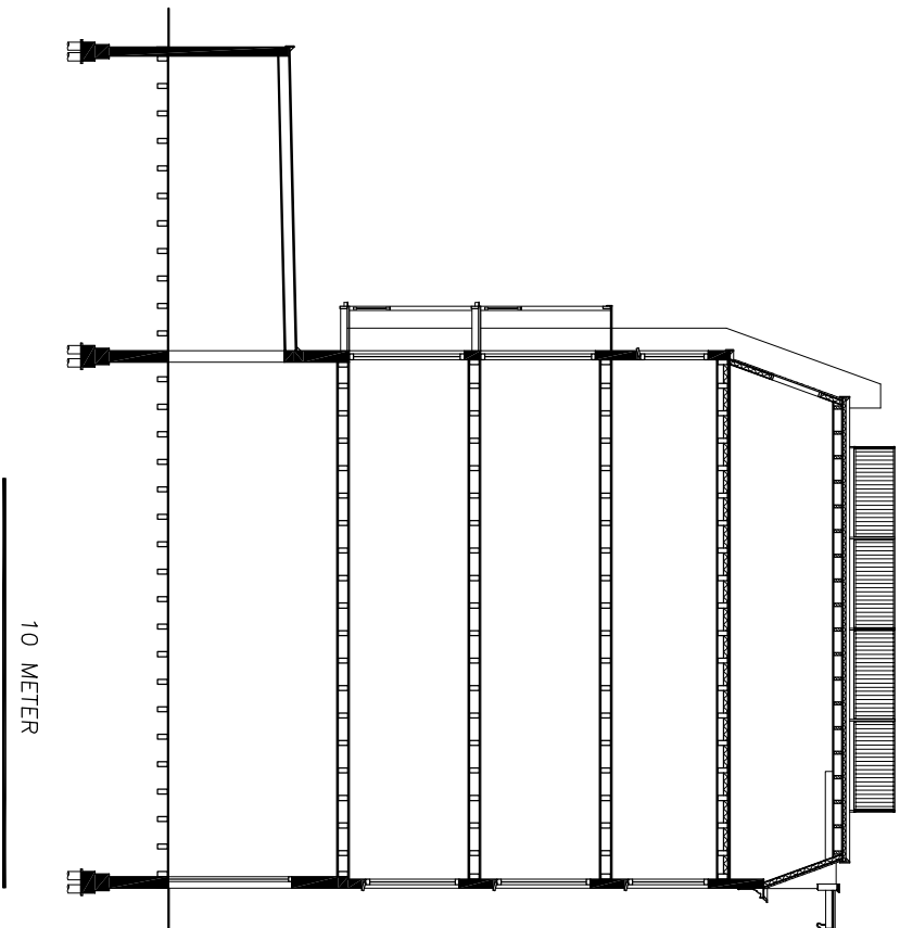
langdoorsnede B-B
