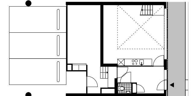
Rijswijkstraat, type B2 BG en 1e verdieping
