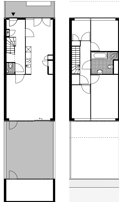
Kwintsheulstraat, type C1 Bg en 1e verdieping
