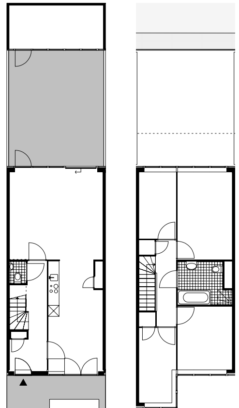
Loosduinenstraat, type A1 BG en 1e verdieping
