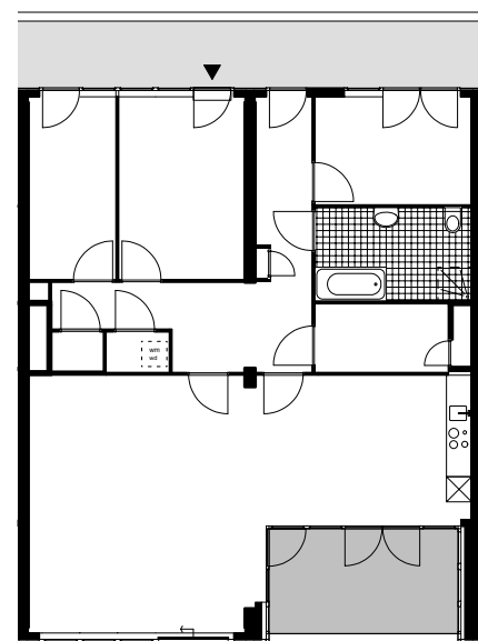
Loosduinenstraat, type A6 4e verdieping
