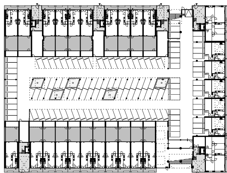
Begane grond
