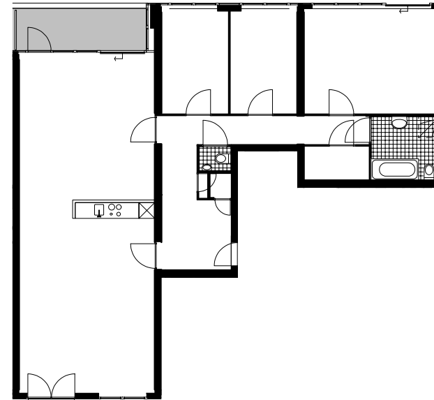
Kwintsheulstraat, type C4 4e verdieping
