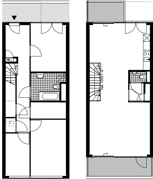
Loosduinenstraat 2e en 3e verdieping
