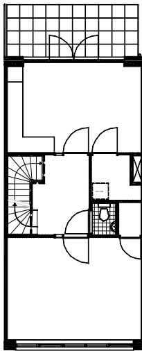
eerste verdieping
