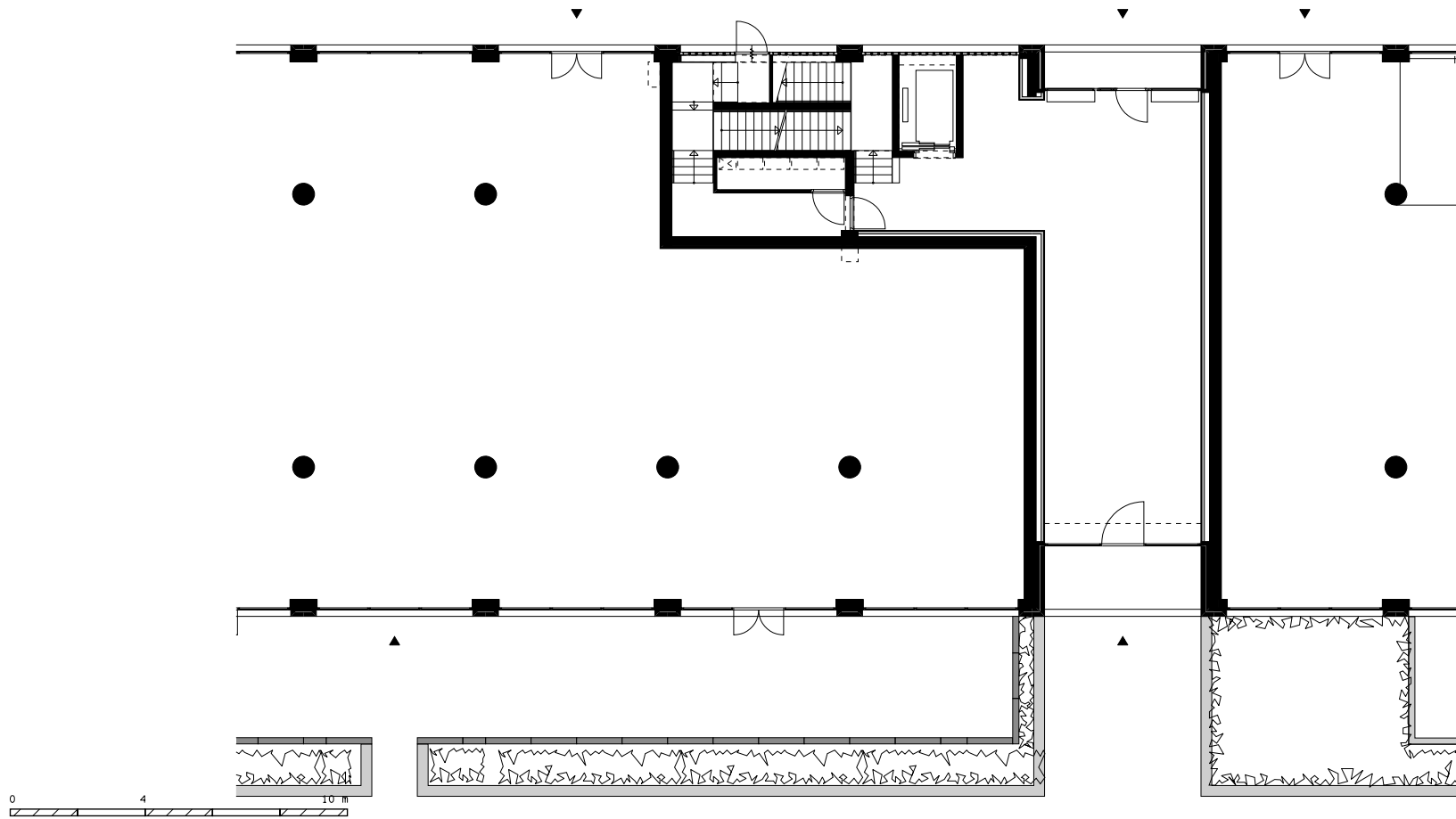
overzicht blok A3, laag 01, entree en commerciële ruimte
