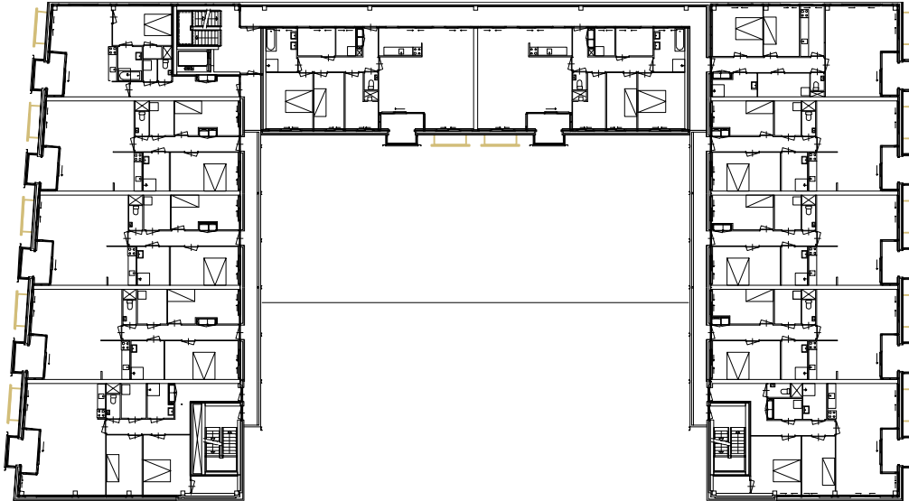
3e VERDIEPING
