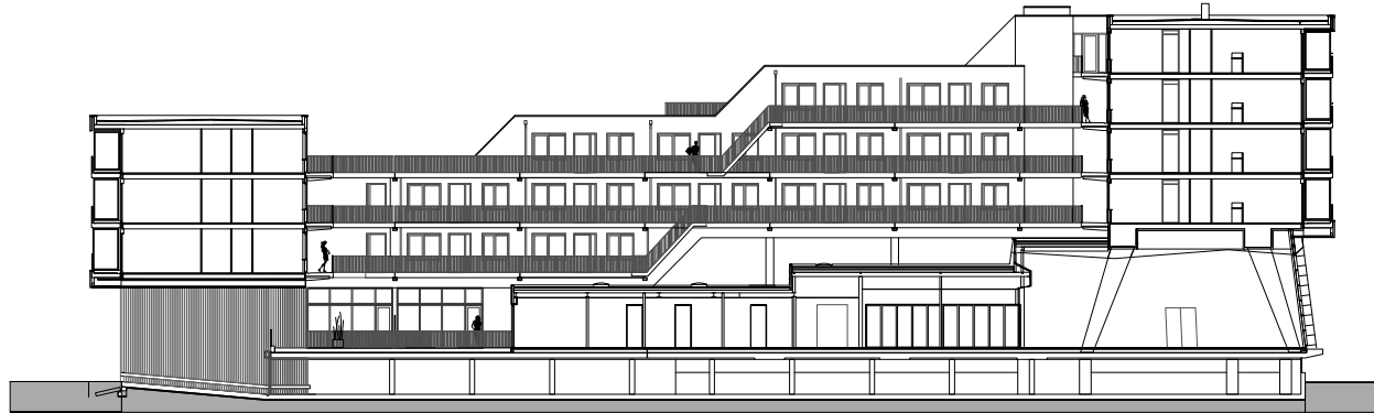
Doorsnede: A-A
