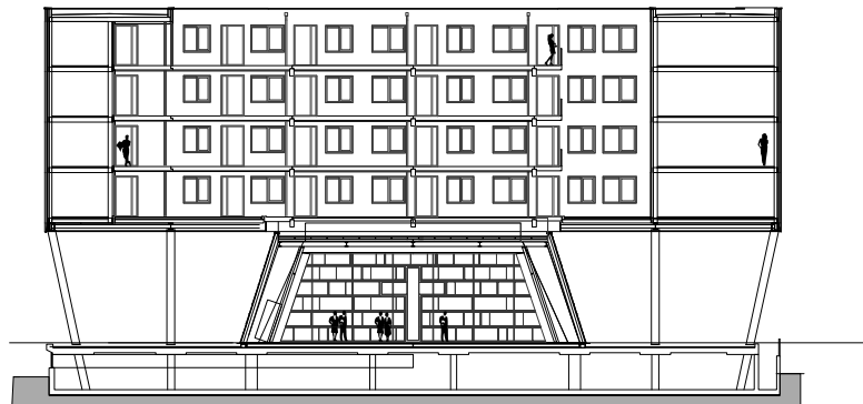
Doorsnede: Be-Be
