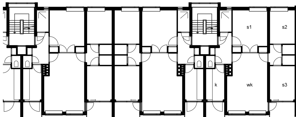
portiekwoningen blok A1 (koop, oorspronkelijke indeling gehandhaafd)
