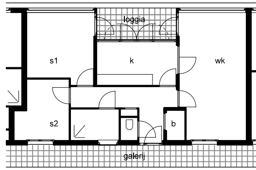
dakwoning galerijblok B1 (Wibo)
