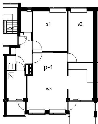
portiekwoningen blok B1 (huur, herindeling)
