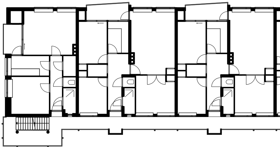
galerijwoningen blok A1 (koop, oorspronkelijke indeling gehandhaafd)
