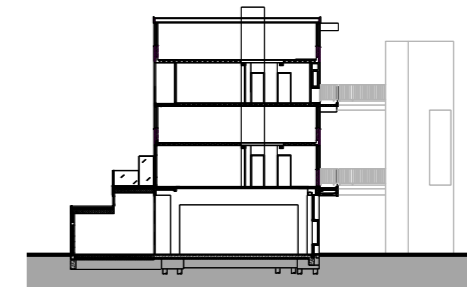
DWARSDOORSNEDE
