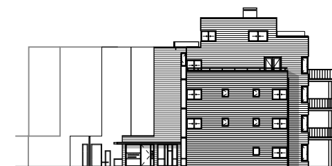
WESTGEVEL HUURWONINGEN
