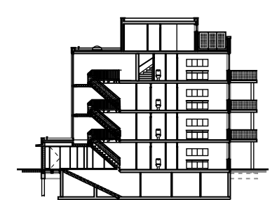
DOORSNEDE A
