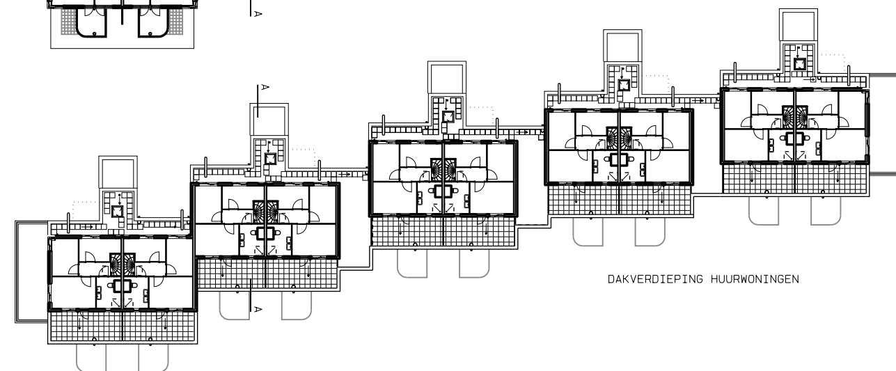
PLATTEGROND 1E/2E VERDIEPING HUURWONINGEN
