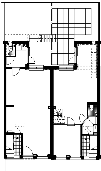
BEGANE GROND TEN KATESTRAAT 39-41
