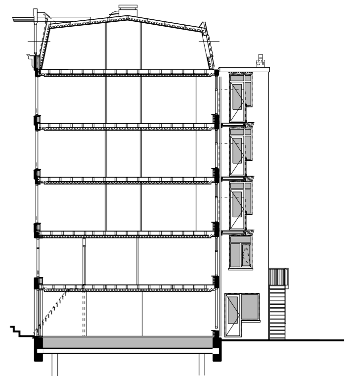
DOORSNEDE TEN KATESTRAAT 39-41
