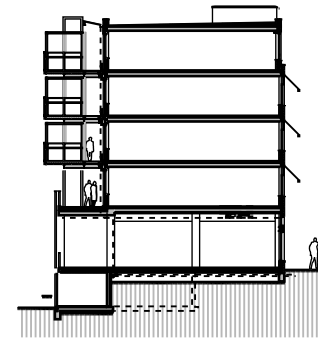
Dwarsdoorsnede Postjesweg
