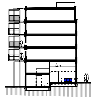
Dwarsdoorsnede Witte de withstraat
