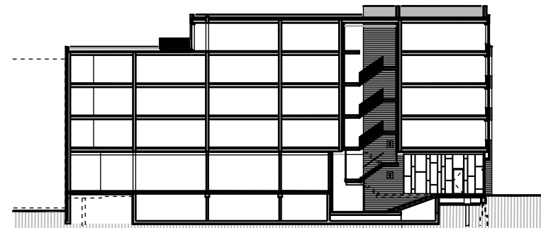
Langsdoorsnede Postjesweg
