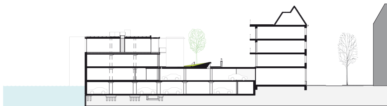
DOORSNEDE A (over deel A (boekbinderij), binnenterrein en garage)
