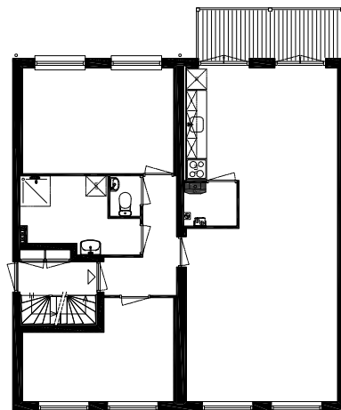
Woningtype A 10 meter
