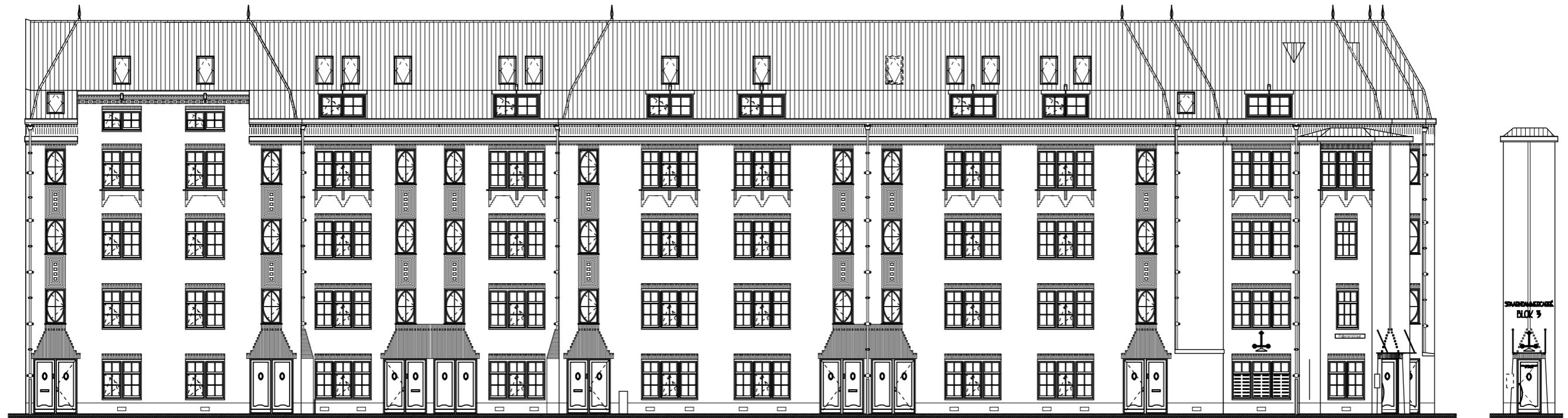
VOORGEVEL POLANENSTRAAT
