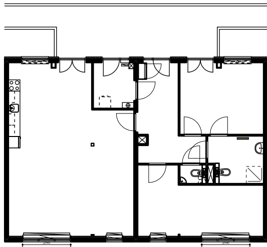
POLANENSTRAAT 1e verdieping
