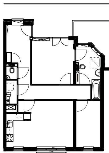
KNOLLENDAMSTRAAT 2e verdieping
