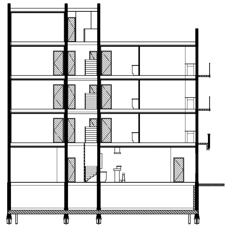
DOORSNEDE D - D
