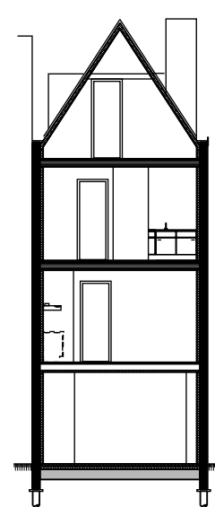
DWARSDOORSNEDE
