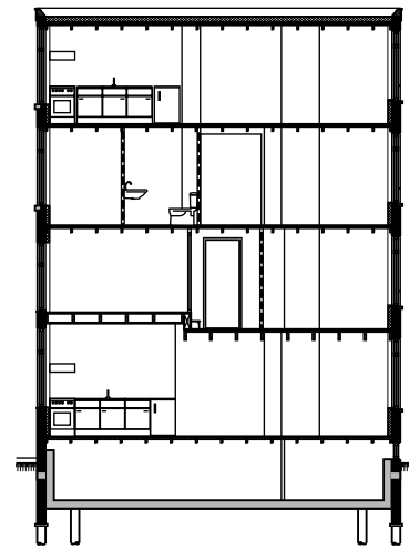
LANGSDOORSNEDE
