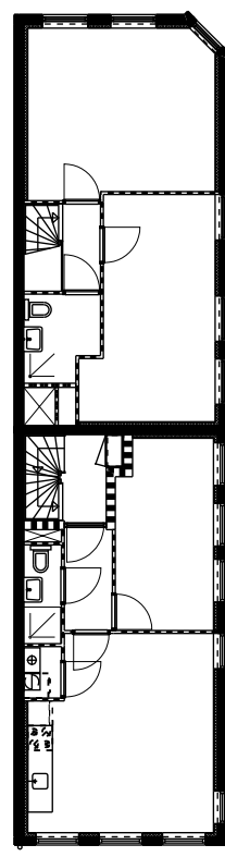
1e VERDIEPING
