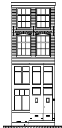
VOORGEVEL
