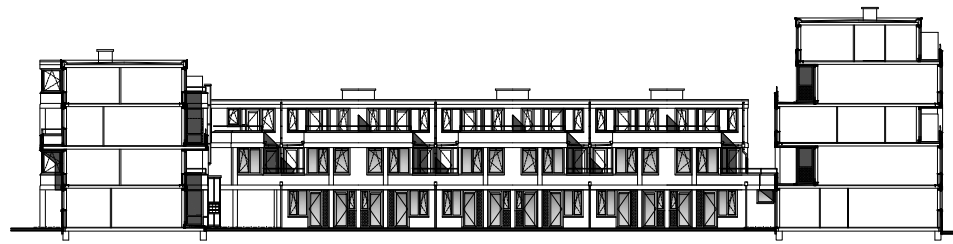
Doorsnede blok A4
