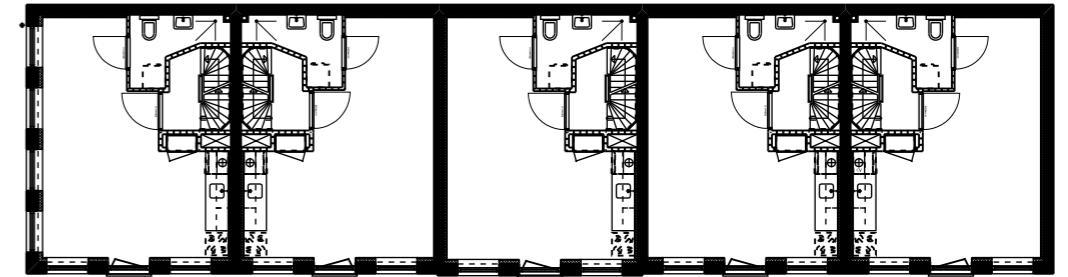
1e, 2e & 3e VERDIEPING
