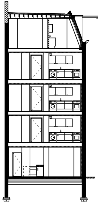
DOORSNEDE
