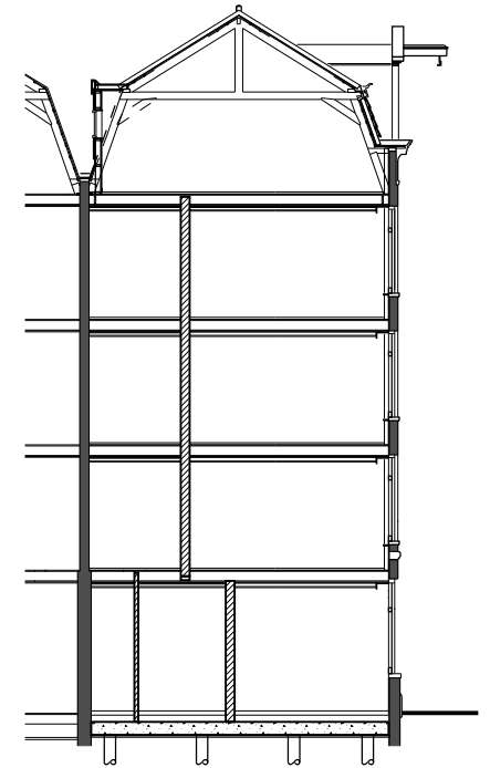
doorsnede
