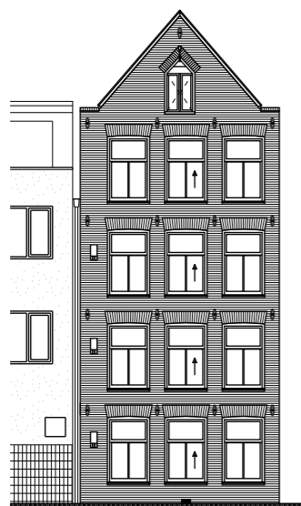
14a Zijgevel
