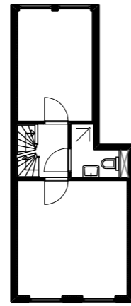
1e VERDIEPING
