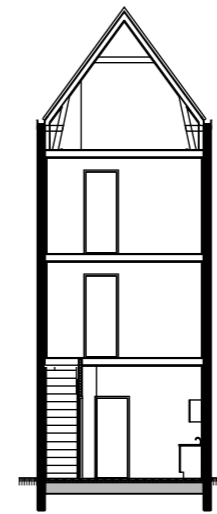
DWARSDOORSNEDE
