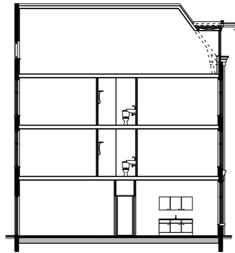
LANGSDOORSNEDE
