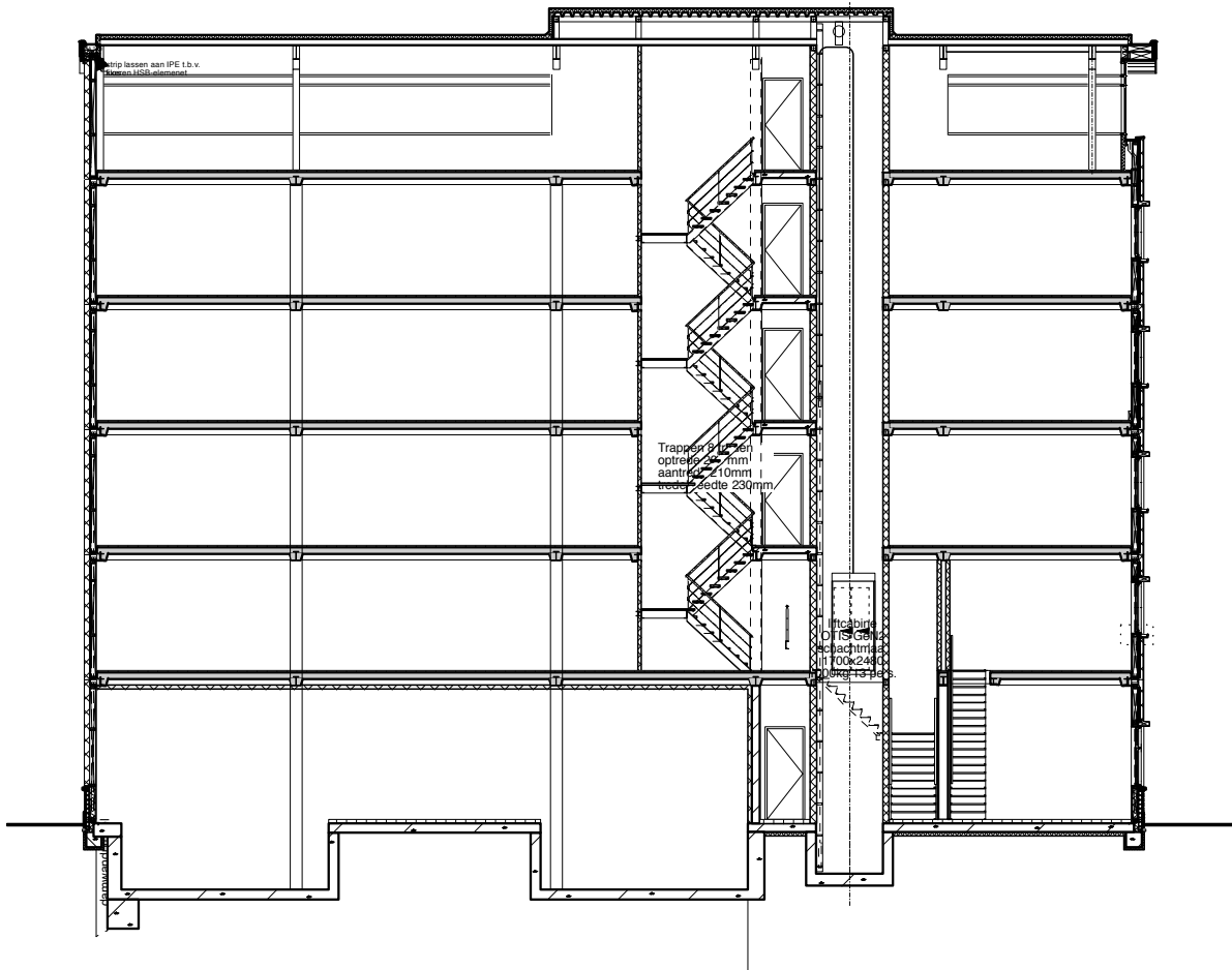
Langs- en dwarsdoorsnede 1:200
