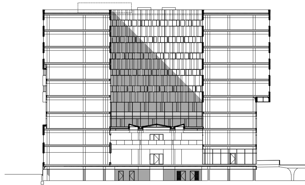
Miro doorsnede
