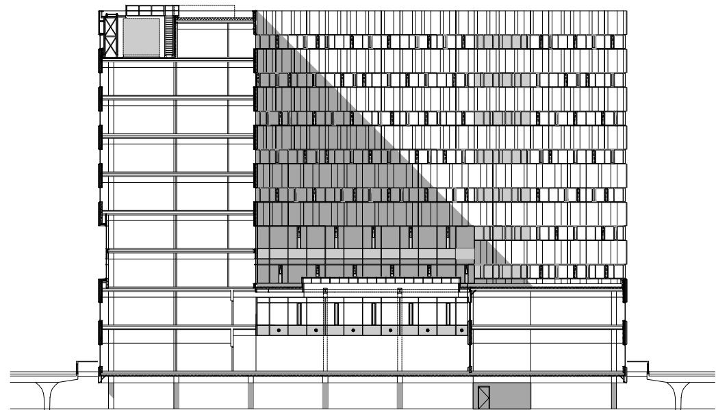
Miro doorsnede
