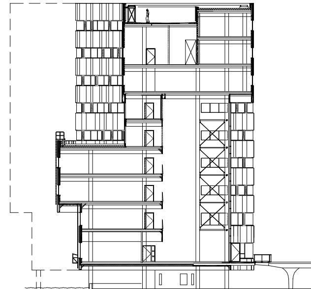
Gaudi doorsnede
