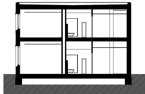
DOORSNEDE C-C
