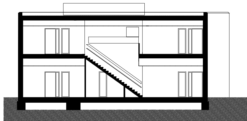
DOORSNEDE B-B
