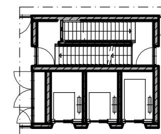
kern 8e verdieping
