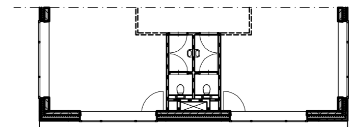
Kopgevel 6e t/m 8e verdieping
