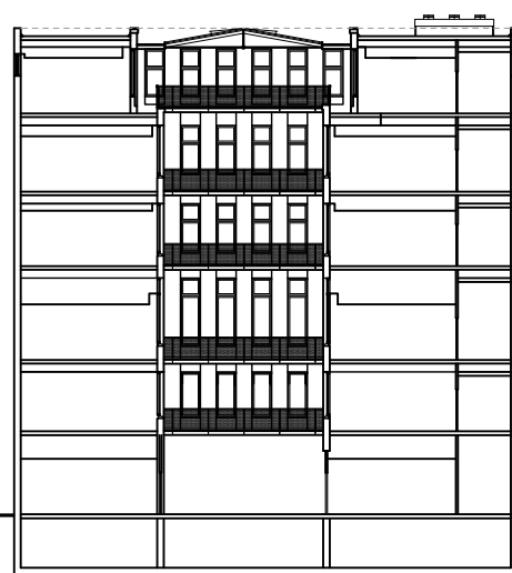
Dwarsdoorsnede
