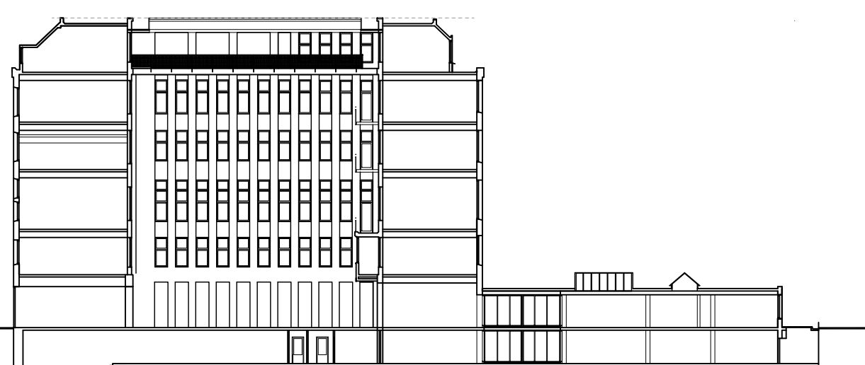
Langsdoorsnede
