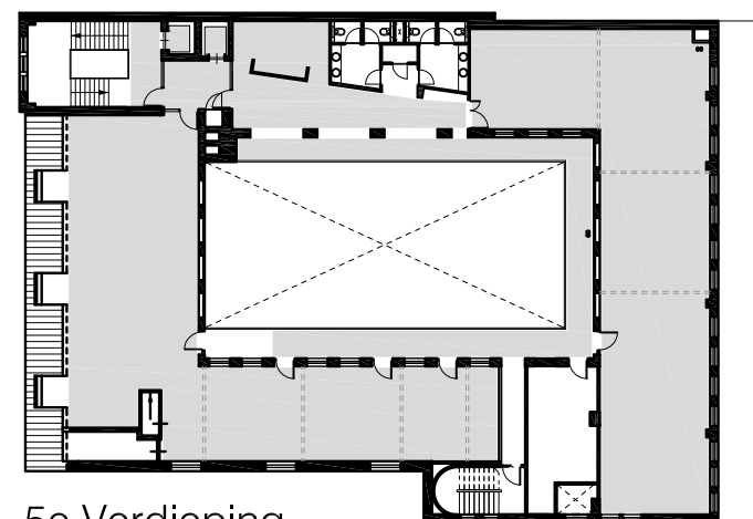
5e Verdieping
