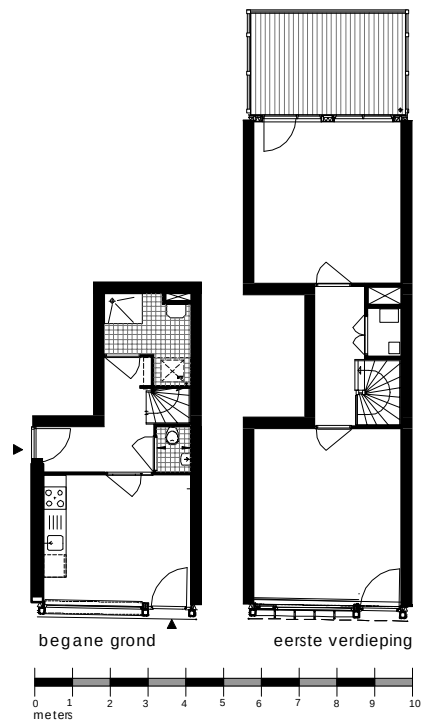
Woningtype 3-A
