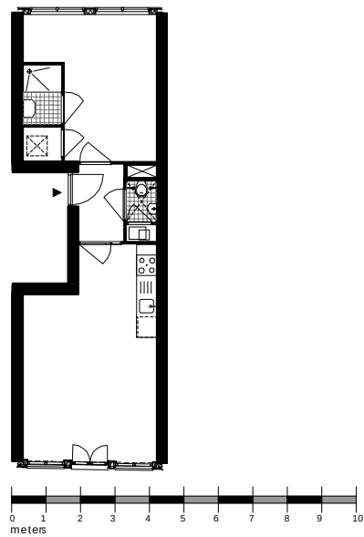
Woningtype 3-B
