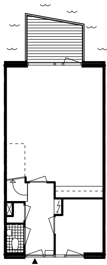
BEGANE GROND
