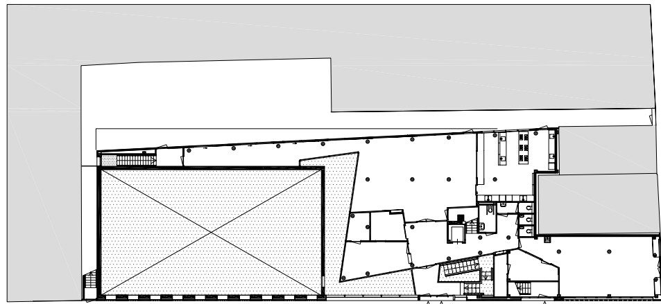
begane grond
