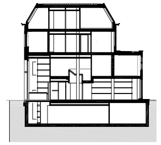
dwarsdoorsnede
