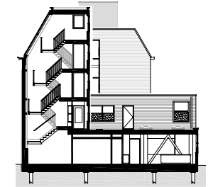
dwarsdoorsnede
