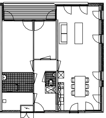
woningtype A (verdieping 1 tm 10)
