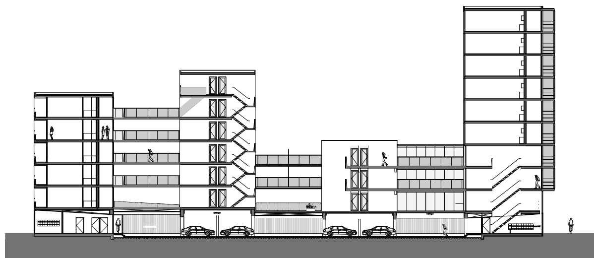
Langs Doorsnede
