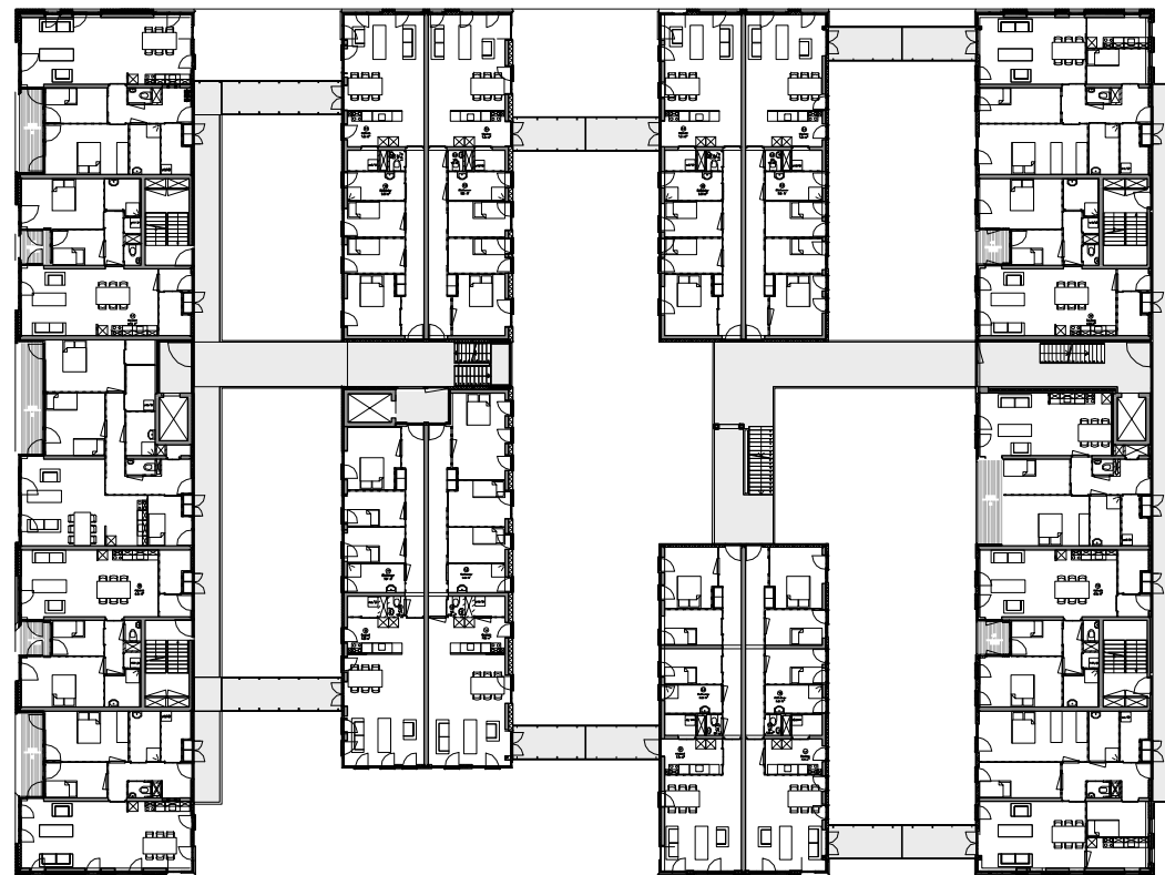
Laag +2
