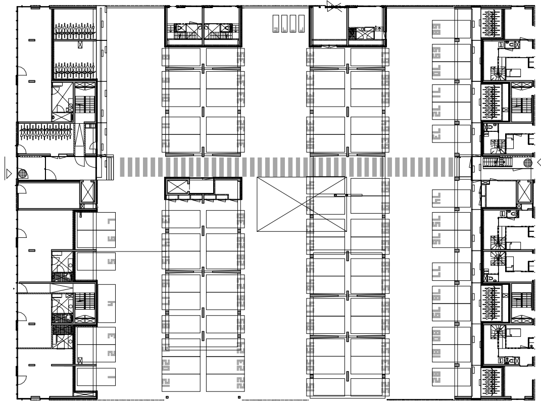
Laag 0
