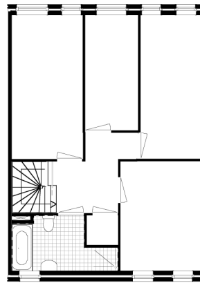
1e verdieping
