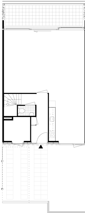
begane grond
