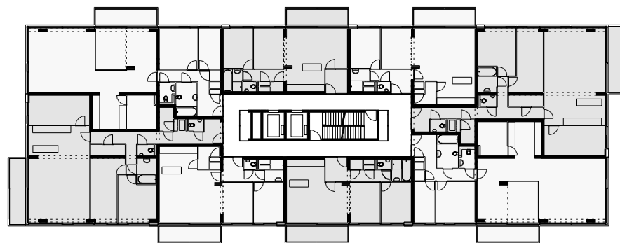
PRINCIPE PLATTEGROND WONINGEN
