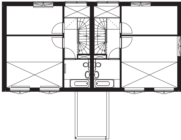
type B eerste verdieping
