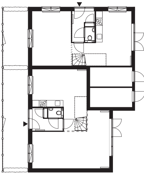
type A bouwnummers 1 en 3
