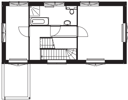
type C eerste verdieping
