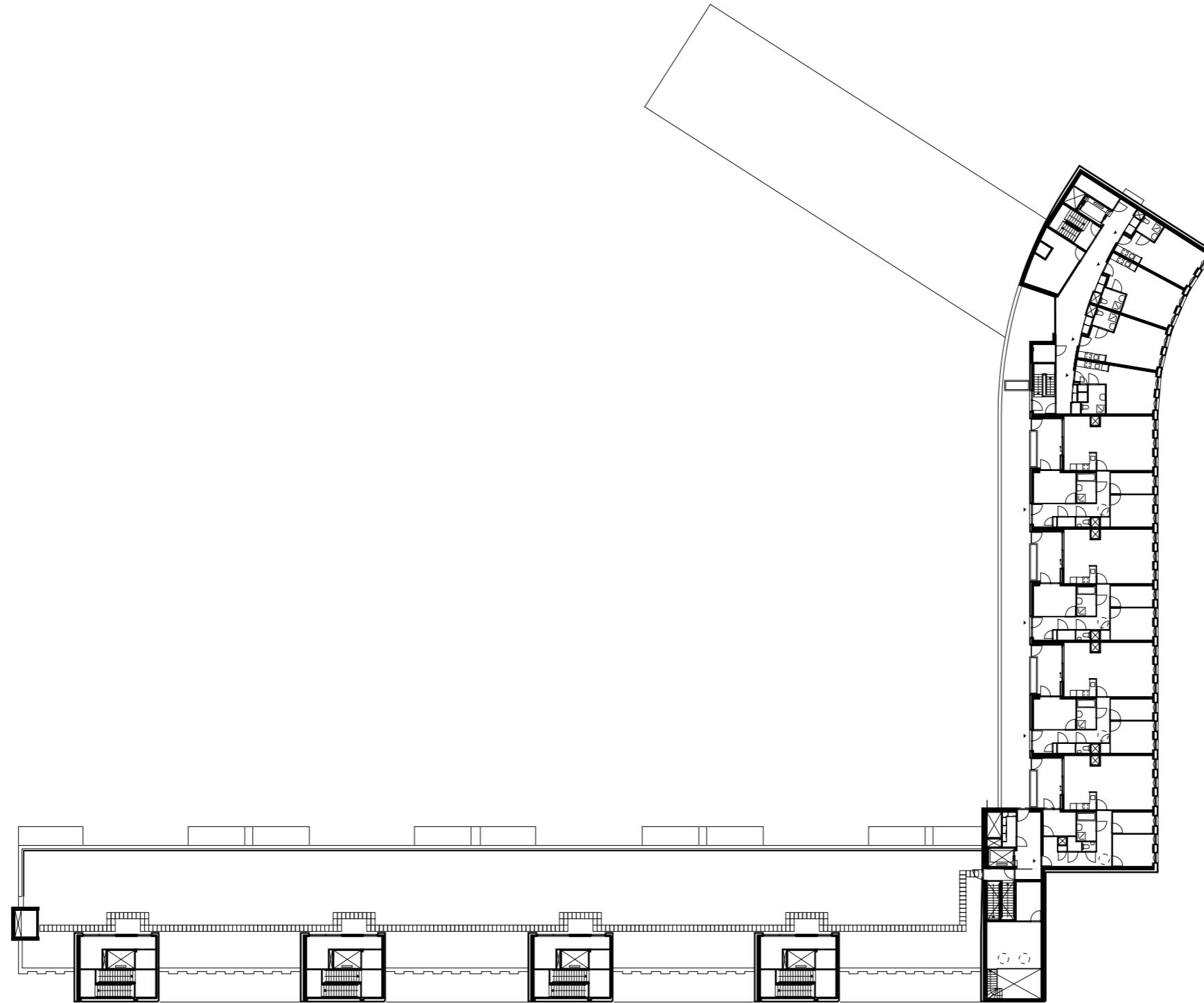
overzichtsplattegrond 8e verdieping
