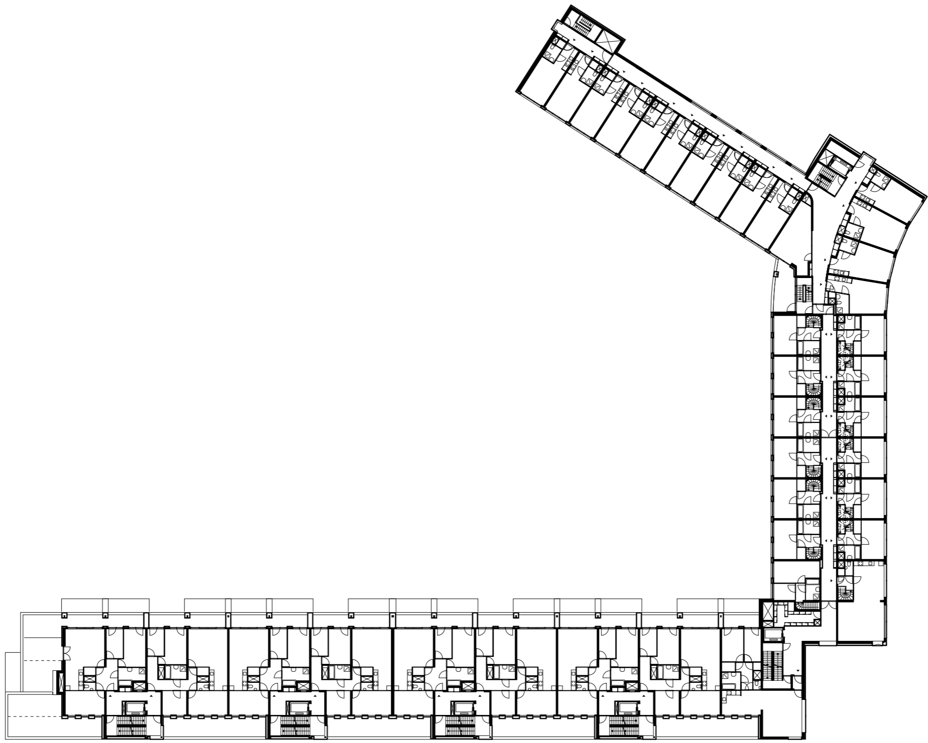
overzichtsplattegrond 6e verdieping
