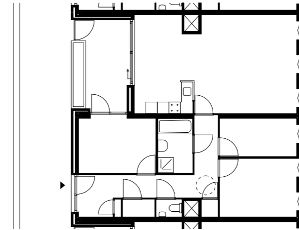
plattegrond 8e verdieping
