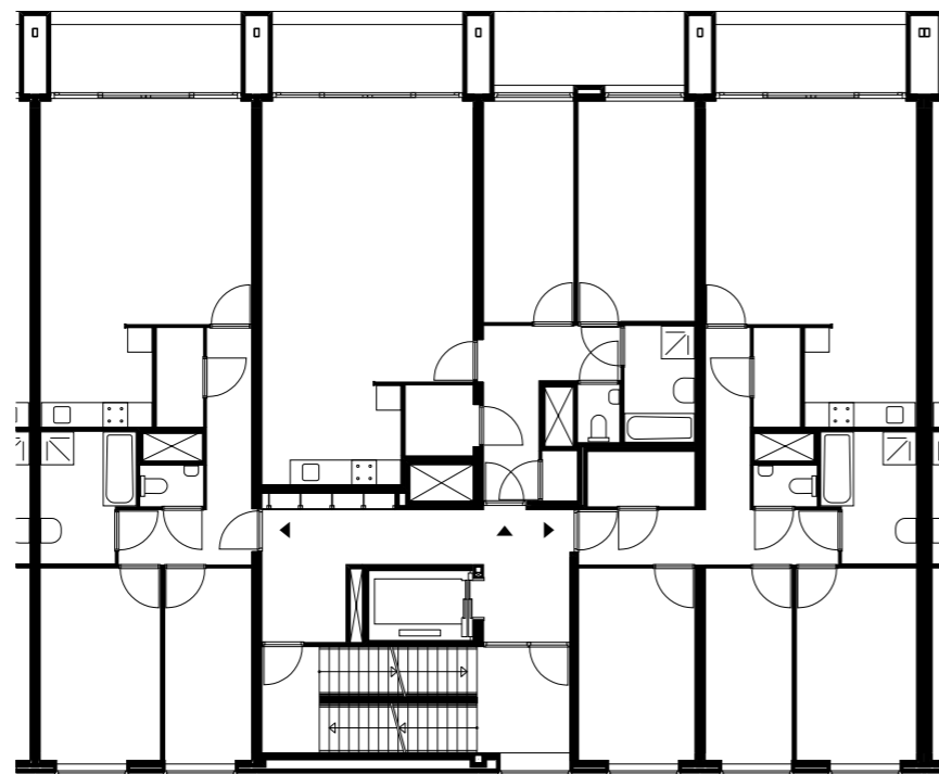
plattegrond 1e tot en met 5e verdieping
