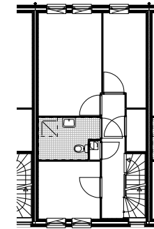
1e VERDIEPING
