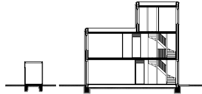
DOORSNEDE
