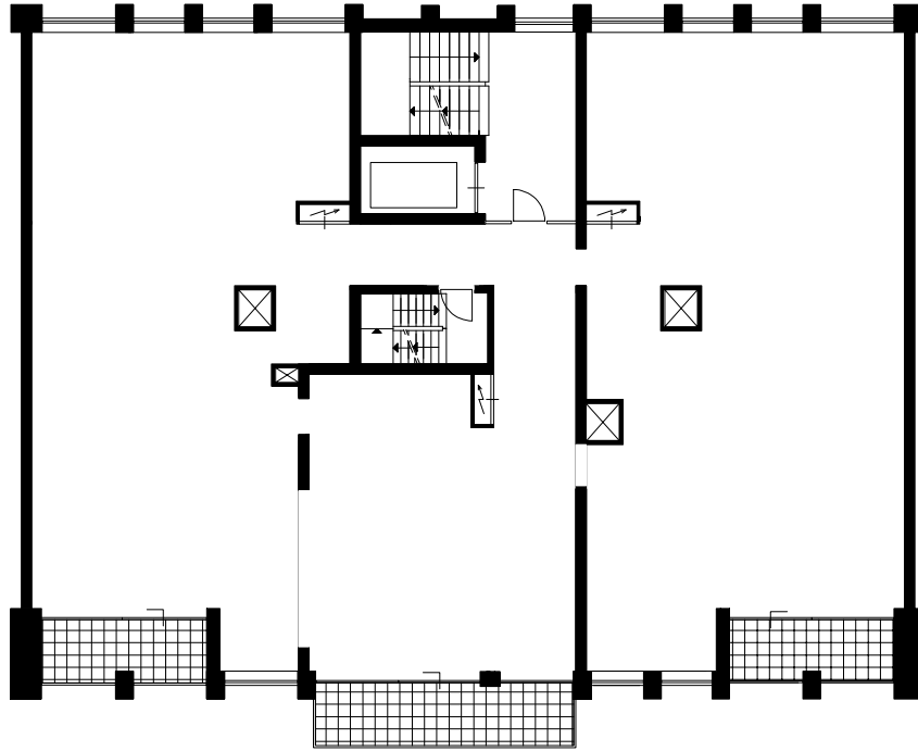
Indelingsvariant 1 Blok 56a IJburg, Amsterdam
