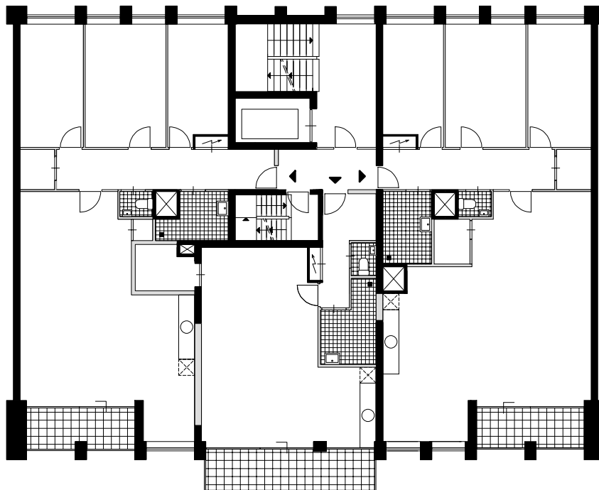
Indelingsvariant 3 Blok 56a IJburg, Amsterdam
