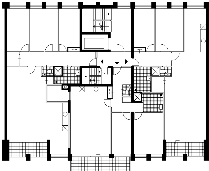
Indelingsvariant 2 Blok 56a IJburg, Amsterdam
