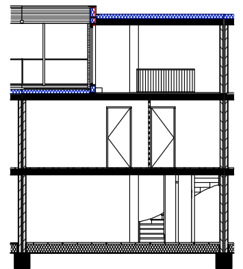
doorsnede
