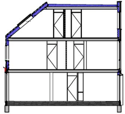
doorsnede
