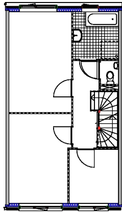
1e verdieping
