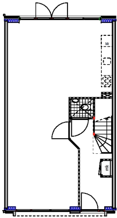
begane grond
