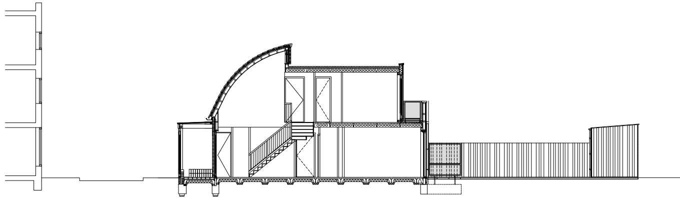
DOORSNEDE 1:200
