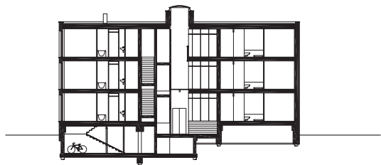
doorsnede B-B
