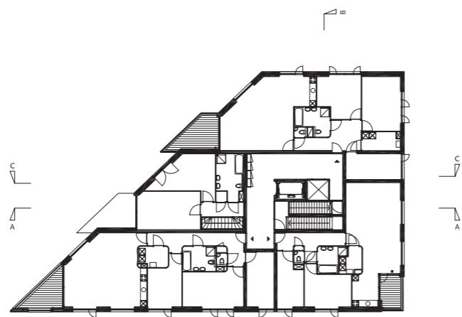
2e verdieping
