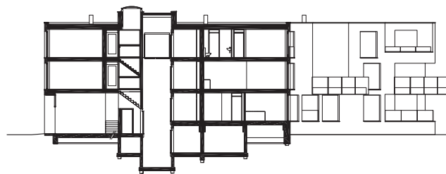
doorsnede C-C
