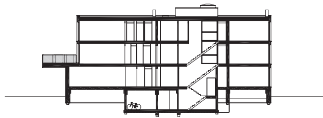
doorsnede A-A
