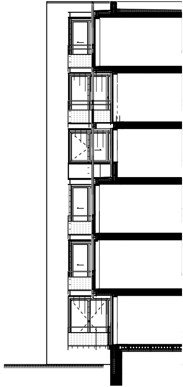
DOORSNEDE
