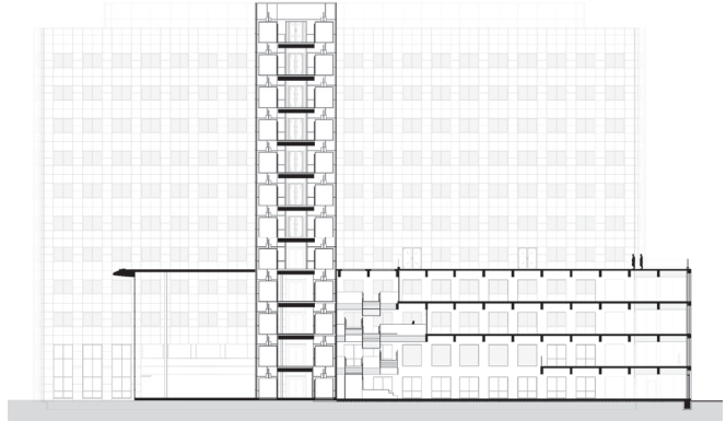
doorsnede
