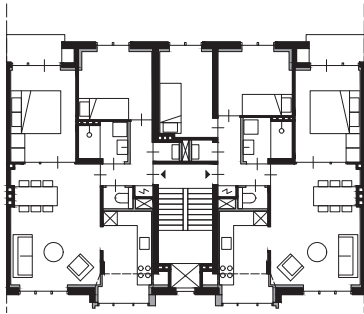
portieketagewoning
