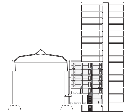
doorsnede
