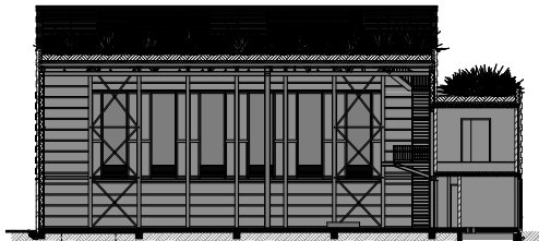
doorsnede
