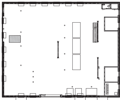
plattegrond
